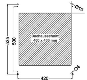
Lochmaß Plisseerahmen
